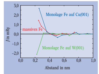
Abb. 2: Rechnungen zur Stärke J der Austauschwechselwirkung zeigen, dass diese für eine Fe-Monolage auf W(001) [4] bei kleinen Abständen negativ ist und die Momente daher antiferromagnetisch ordnen. Im Gegensatz dazu ist J für massives Eisen [2] oder eine Fe-Monolage auf Cu(001) [3] positiv, sodass diese Systeme ferromagnetisch ordnen. (1 Ry \equiv 13,6 eV)
