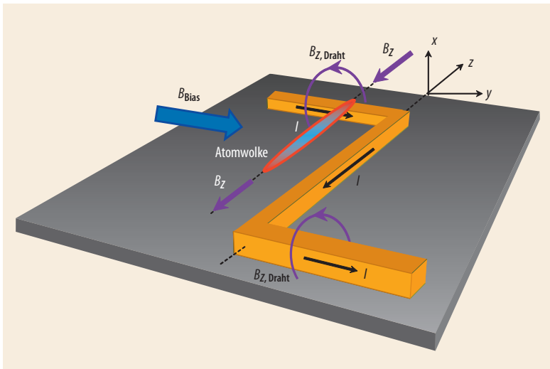
Abb. 1 Ein Z-förmig gebogener Draht erzeugt eine einfache Fallengeometrie für neutrale Atome: In einem magnetischen Minimum über dem Draht sammeln sich die Atome. Die Biegung sorgt für eine zusätzliche Magnetfeldkomponente, die den vollständigen Einschluss in allen Raumrichtungen gewährleistet.
