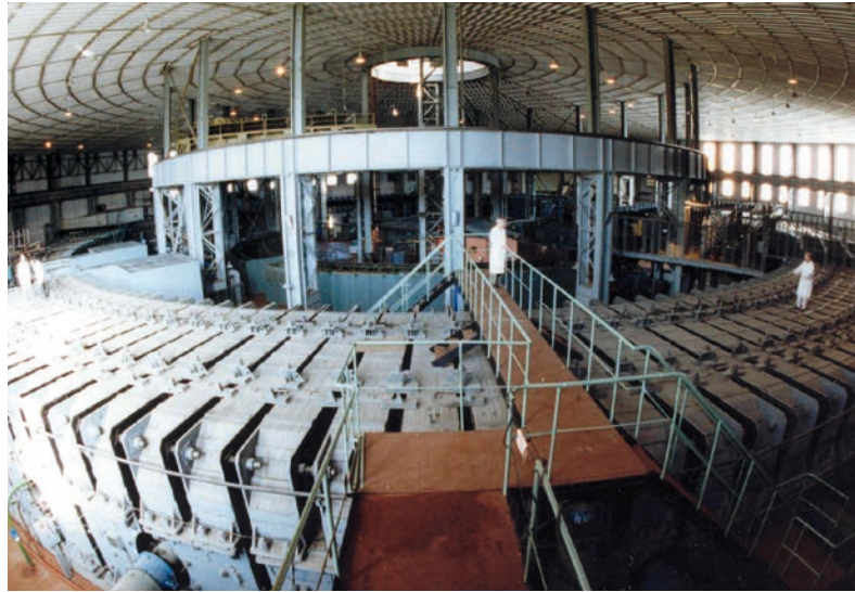
Abb. 4 Das Synchrophasotron beschleunigte Protonen auf Energien bis zu 10 GeV. Der Betrieb wurde 2003 eingestellt – hier entstehen die Vorbeschleuniger von NICA.
